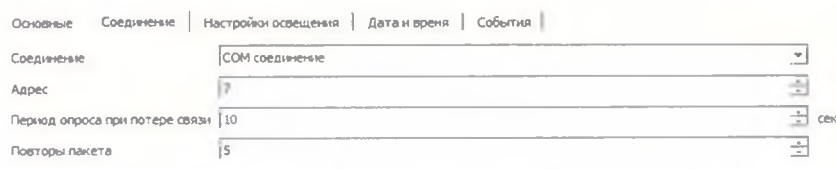
Рисунок 9 – Вкладка «Соединение»
