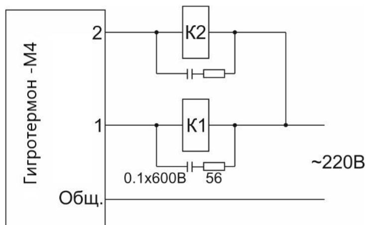
Рисунок 5 – Схема подключения индуктивной нагрузки
